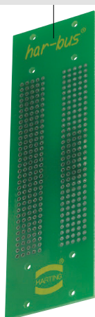
Rückwandplatine (Backplane)
