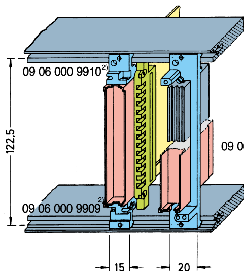
Einzelbefestigung
