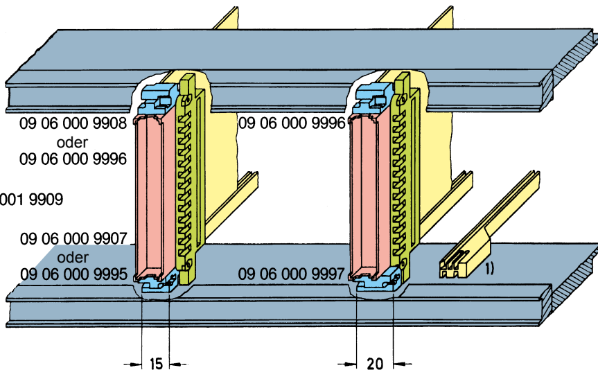
Summenbefestigung
