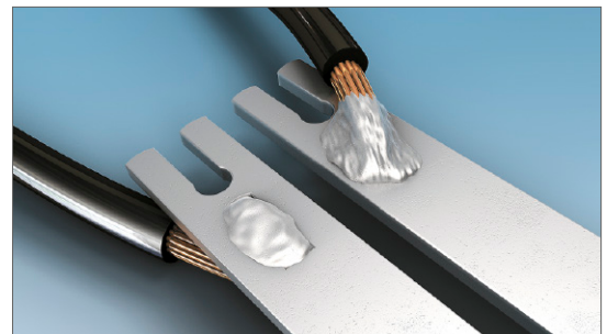
Lötösen-Anschluss
